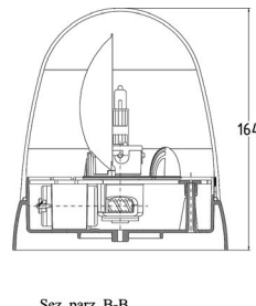
Sez. parz. B-B
