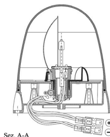
Sez. A-A
